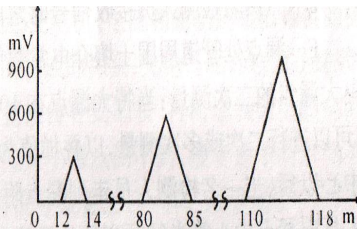
图 15 破损点大小曲线图
