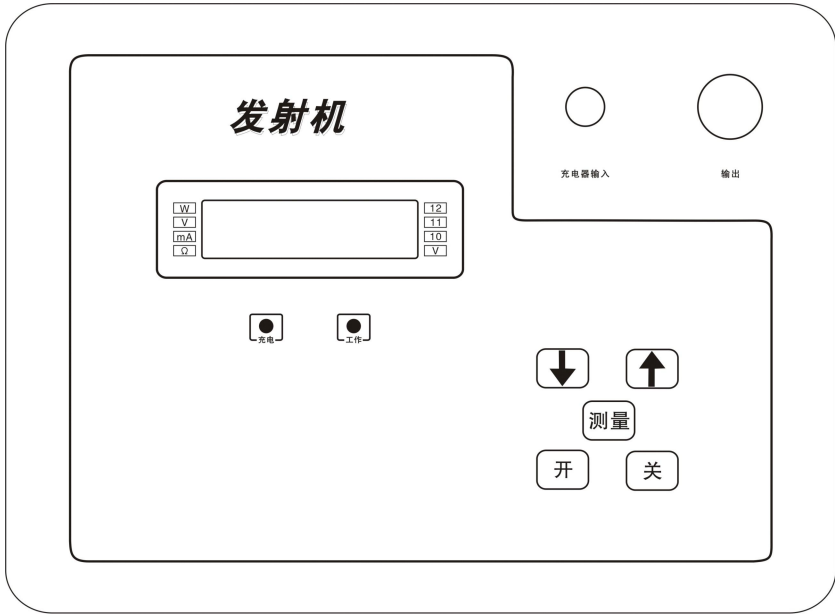
图 1 发射机前面板示意图
