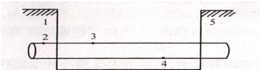
图 17 管道防腐层破损处开挖验证示意图
